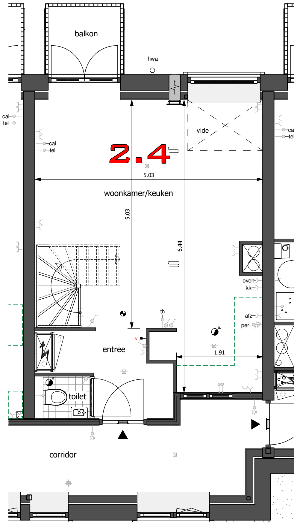
2e verdieping
