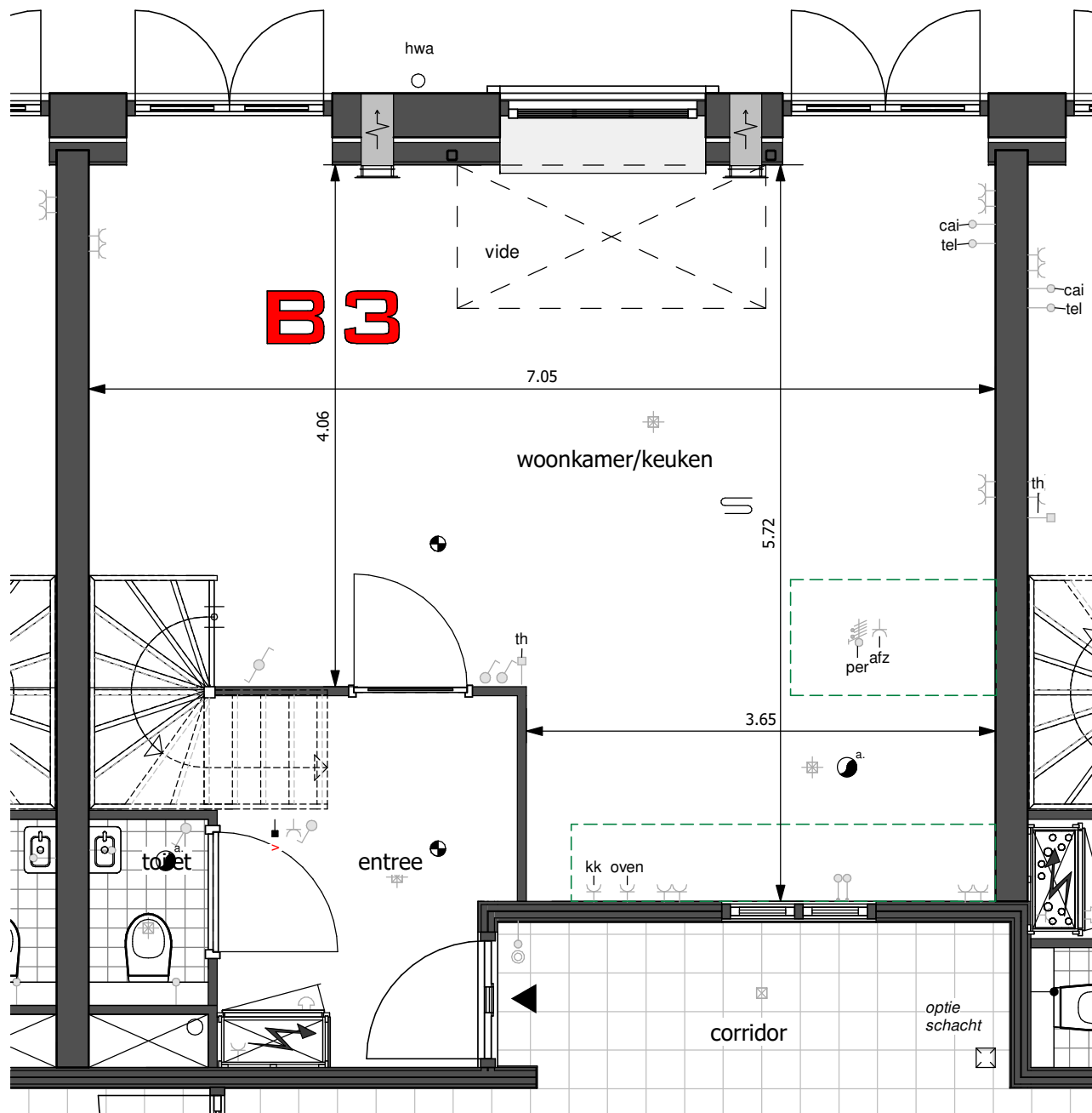
begane grond
